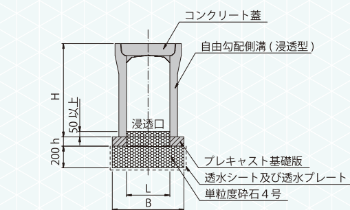
標準（浸水部）断面図
