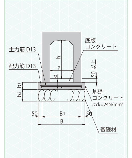
標準施工図
