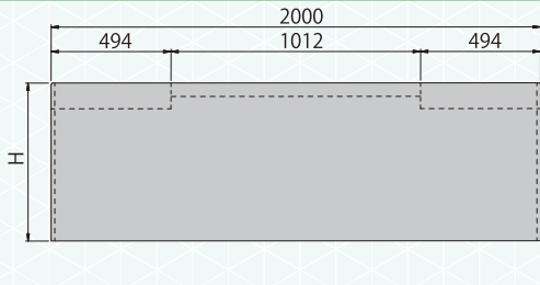
B-B 断面図
