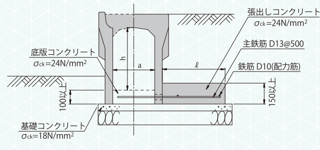
標準施工図
