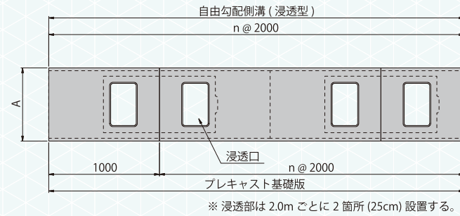
プレキャスト基礎版平面図
