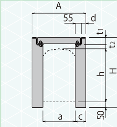
A-A 断面図
