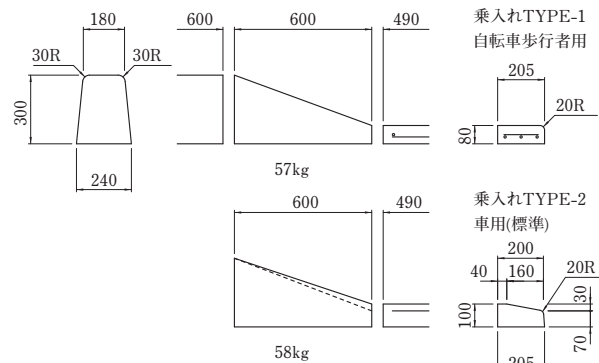
両面歩車道B～FN乗入れ(1本切下げ)
