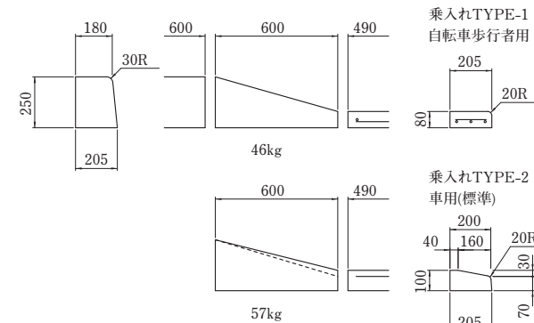
片面歩車道A～FN乗入れ(1本切下げ)
