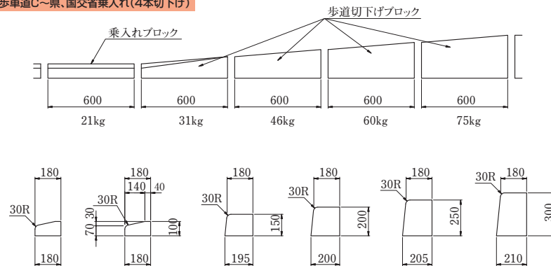
片面歩車道C～県、国交省乗入れ(4本切下げ)
