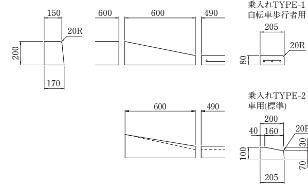
片面歩車道A～FN乗入れ(1本切下げ)
