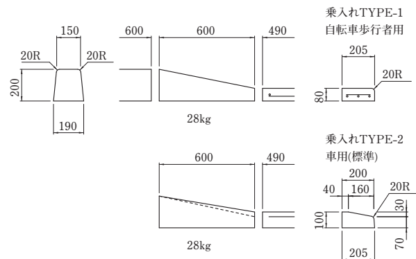
両面歩車道A～FN乗入れ(1本切下げ)
