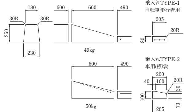
両面歩車道B～FN乗入れ(1本切下げ)
