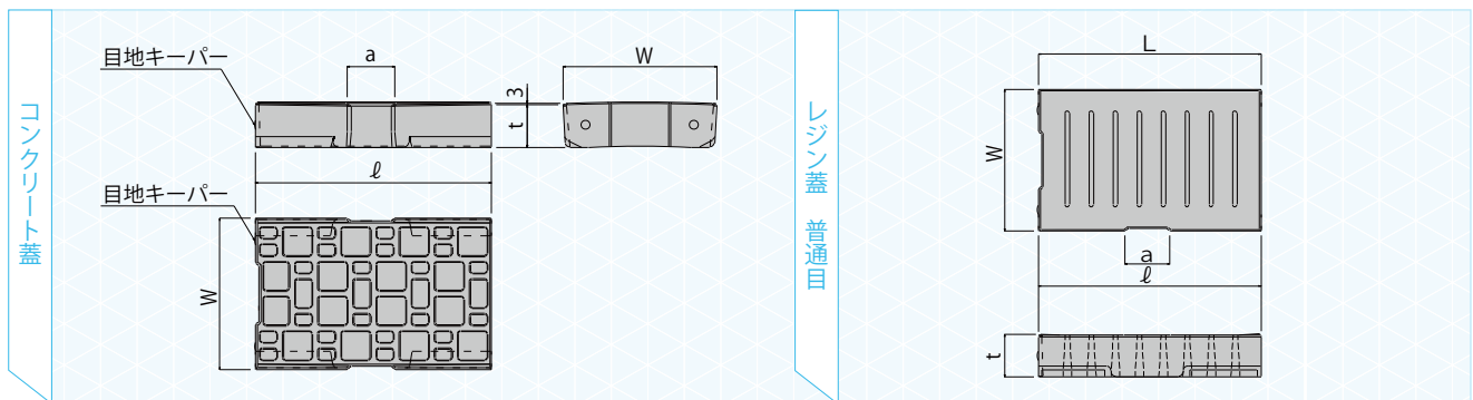
L=1000 タイプ姿図
