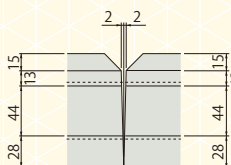
縦目地(突き合わせ)
