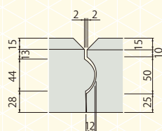
縦目地(突き合わせ)
