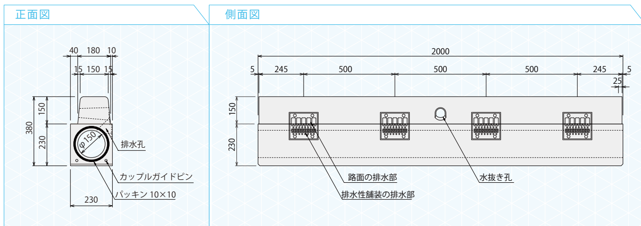
標準タイプ 歩車道境界ブロック A 両面 R 参考重量：279kg
