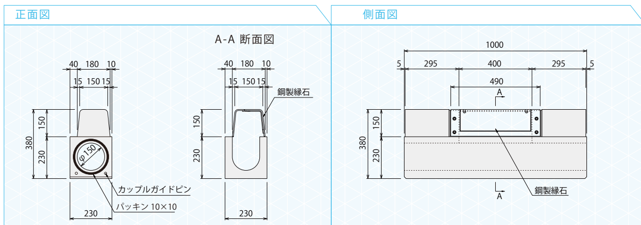
標準タイプ 管理用ブロック 参考重量：115kg
