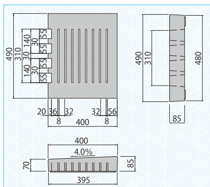
レジン集水蓋 4%
