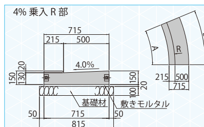
標準施工図
