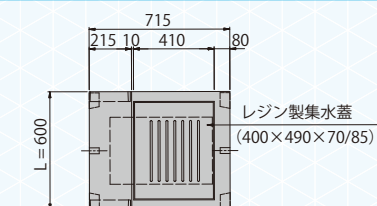
平面図
