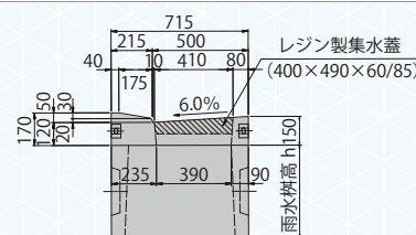
乗入れ4% (A,B タイプ)
